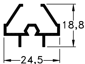
570 - Perimetral peso: 0,20 Kg/m
