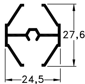
571 - Travesaño peso: 0,27 Kg/m
