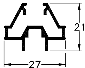
470 - Perimetral peso: 0,27 Kg/m
