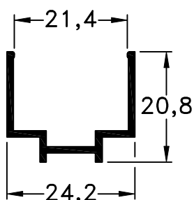
553 - Adaptador D.V.H. peso: 0,21 Kg/m
