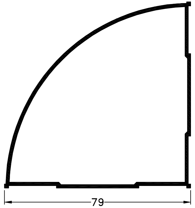
986 - Columna Curva peso: 1,06 Kg/m
