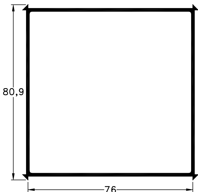
455 - Perfil Columna peso: 1,18 Kg/m
