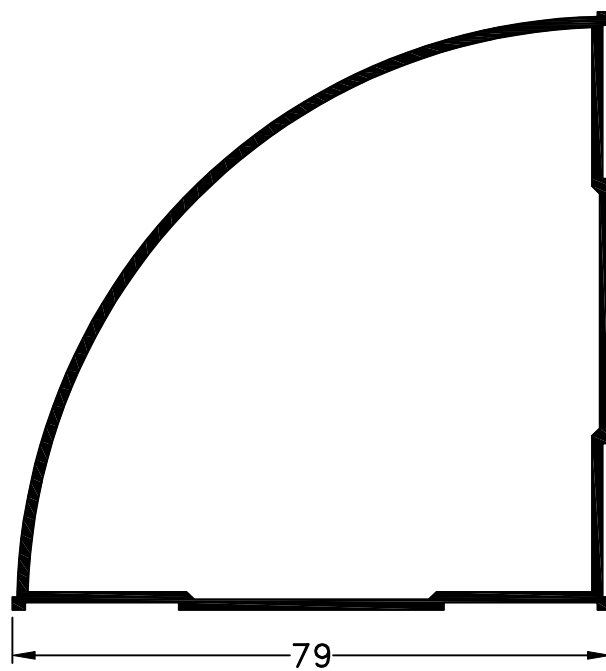
986 - Columna Curva peso: 1,06 Kg/m
