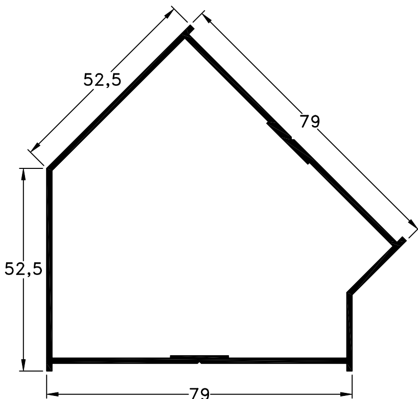
43 - Columna Recta peso: 1,17 Kg/m
