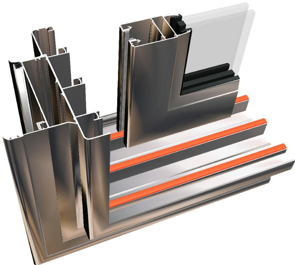
874 - Marco Corrediza de Tres Guías M-Cinco peso: 2300 g/m
